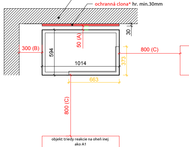
PÔDORYS - umiestnenie pri nehorľavej nosnej priečke. Min. odstup 0 mm.
